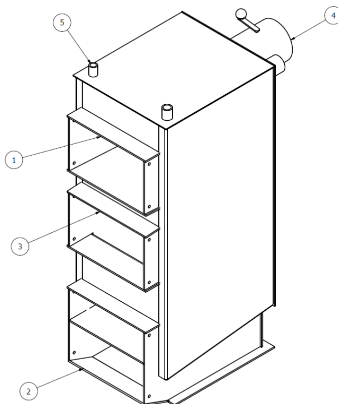
Rys.11. Schemat stalowego korpusu kotła KLIMOSZ IRON.
