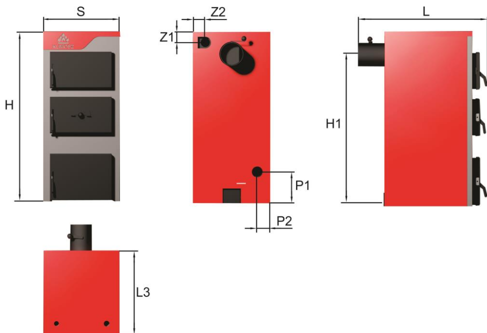
Rys. 13. Wymiary kotłów KLIMOSZ WALLY 26.
