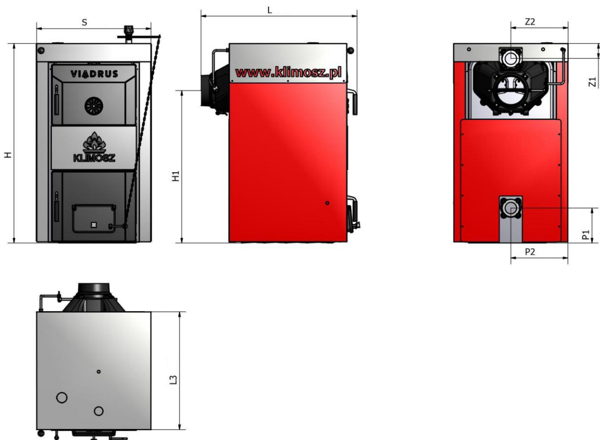
Rys.12. Wymiary kotłów KLIMOSZ WALLY.
