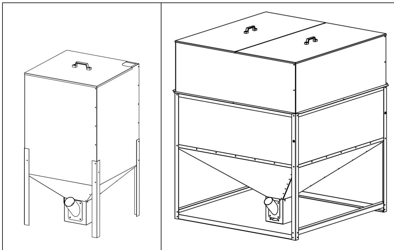
Rys. 26. Rysunek zasobnika paliwa 300 i 900 dm 3 .
