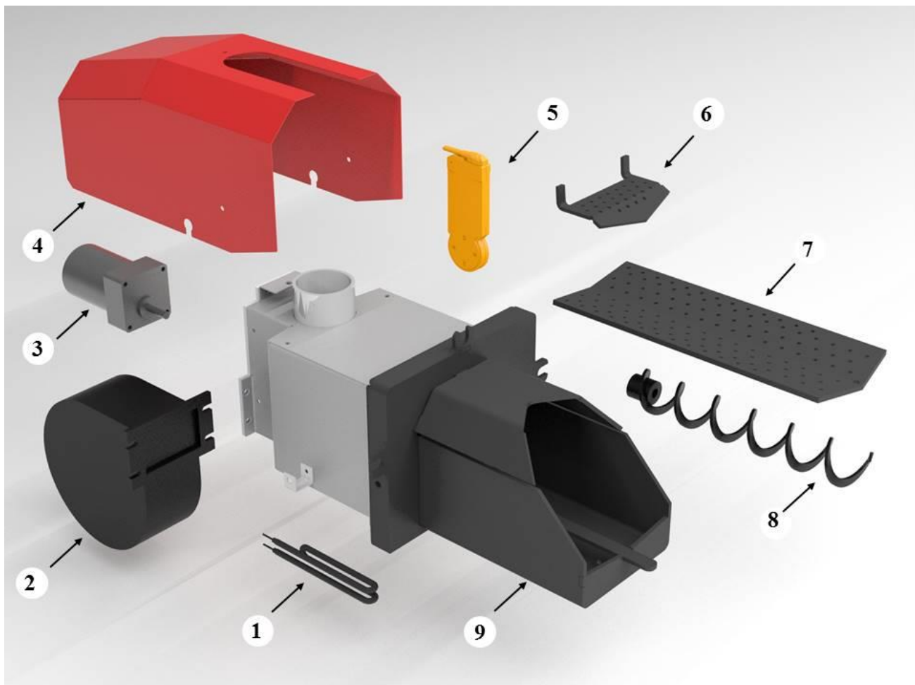
Rys. 20. Schemat ideowy palnika peletowego.
