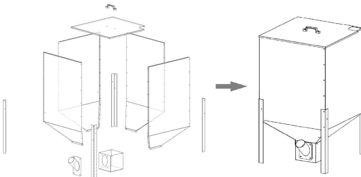
Rys. 25 Montaż zbiornika 300l do zestawu palnika peletowego.
