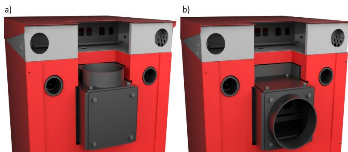
Rys. 17. Montaż króćca czopucha w kotłach KLIMOSZ DUOPELET NG/EKO a) pozycja pionowa b) pozycja pozioma.
