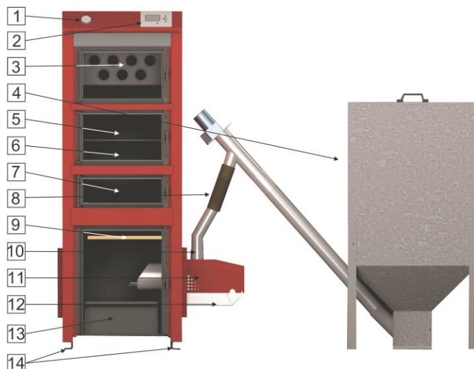
Rys. 23. Opis kotła KLIMOSZ DUOPELET (na przykładzie kotła w wersji NG).
