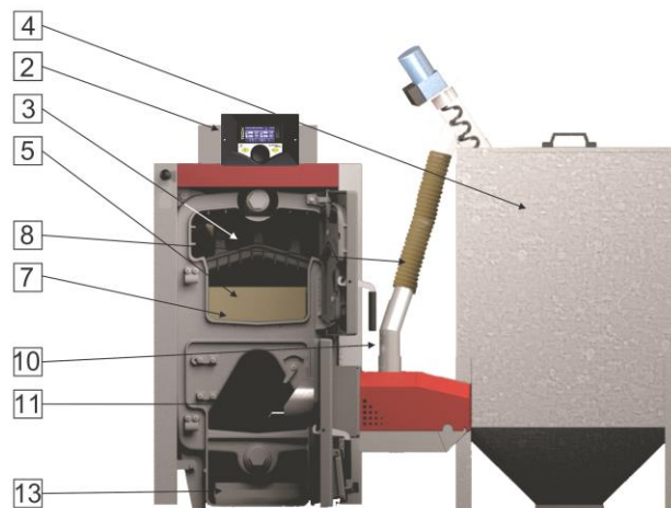
Rys. 24. Opis kotła KLIMOSZ UNIPELET.
