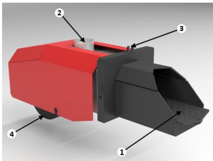
Rys.19. Palnik peletowy.
