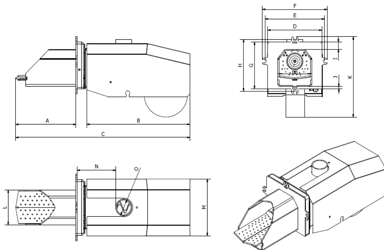
Rys. 21. Wymiary palnika peletowego.
